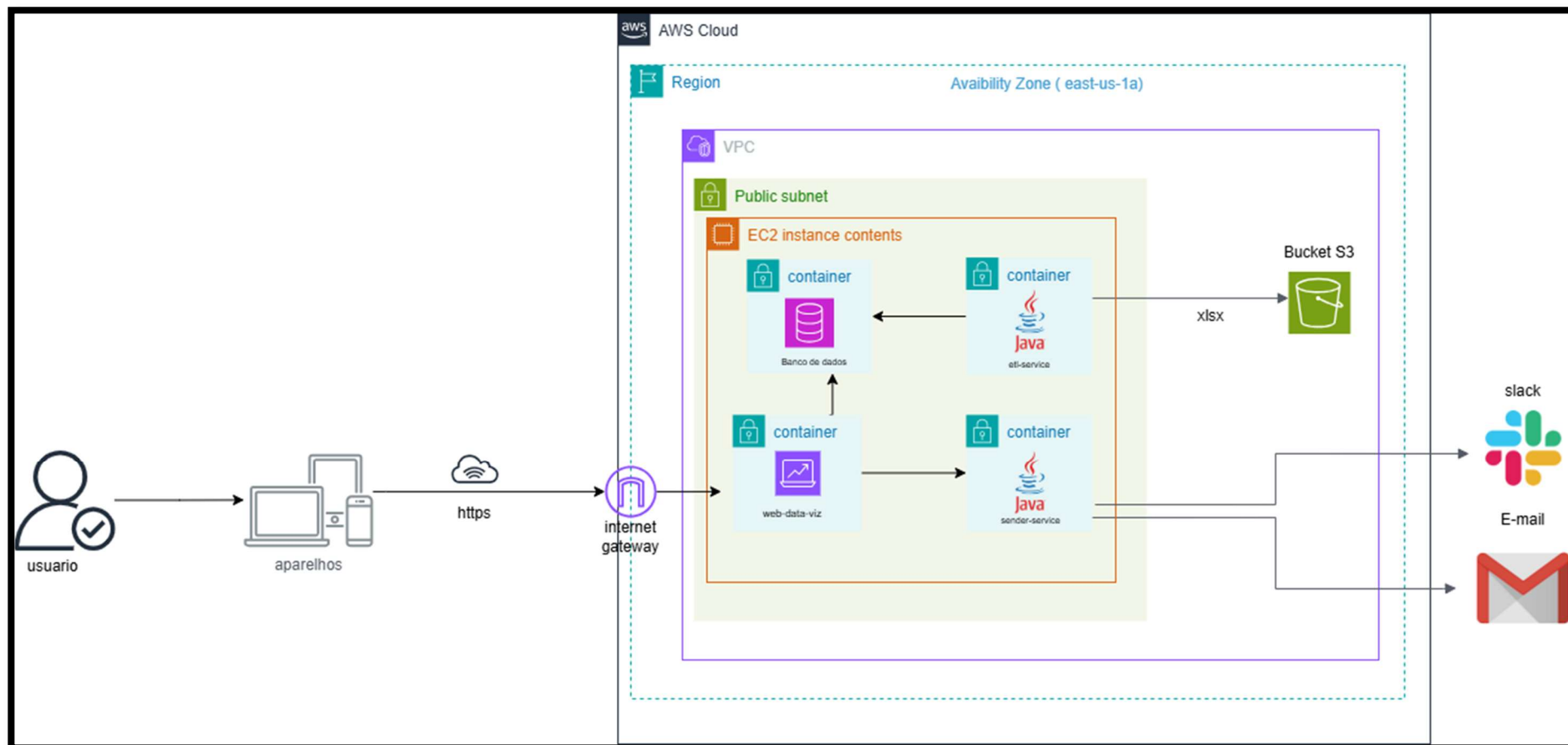
Figura 31 – Arquitetura da Solução da Safety Intelligence.
